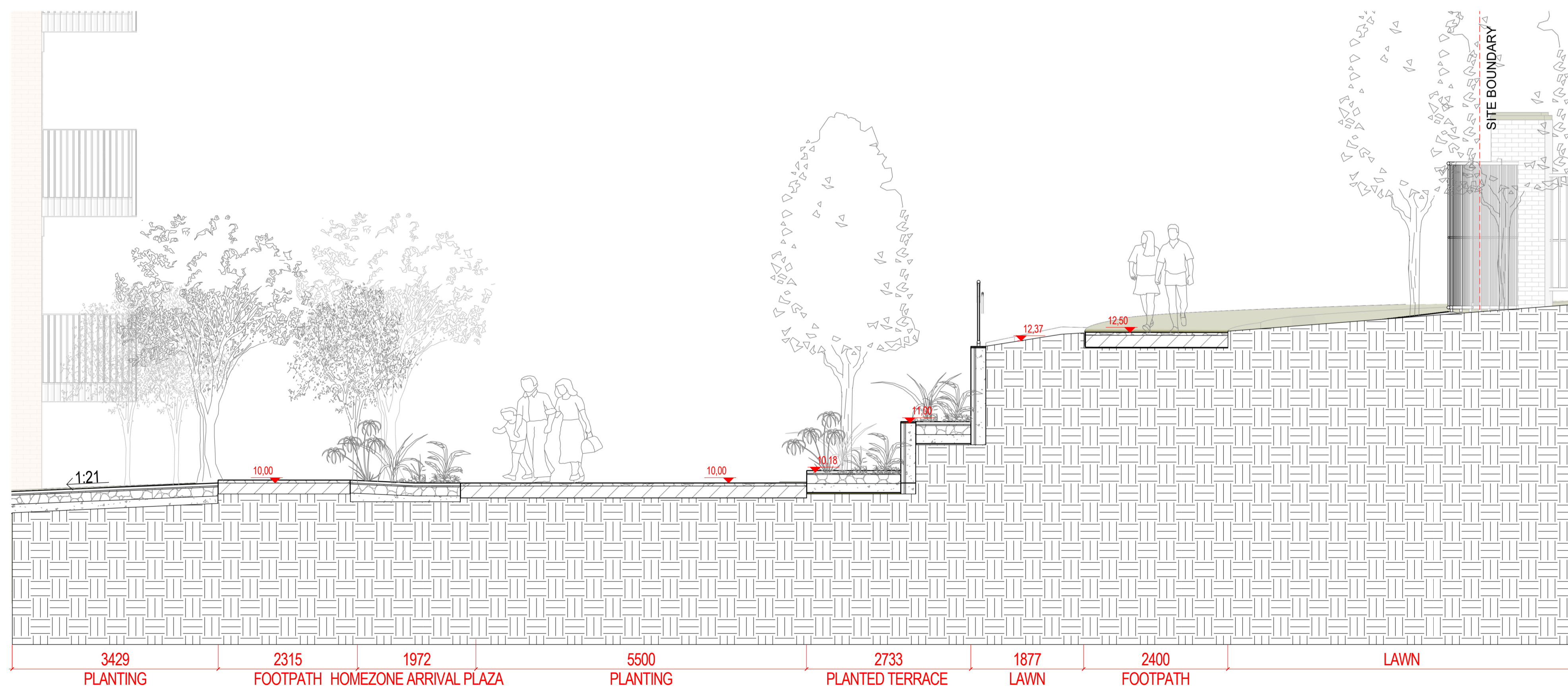
2 SECTION 57 1:50 @A1
