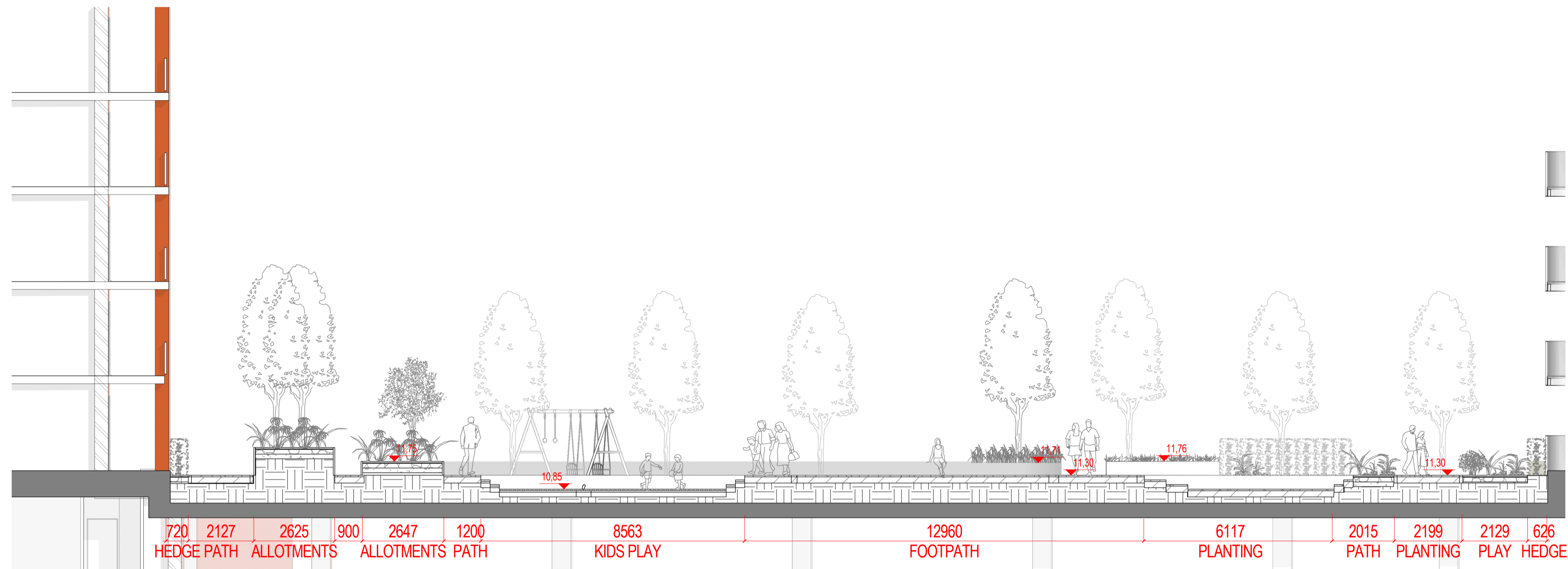
1 SECTION 56 1:100 @A1
